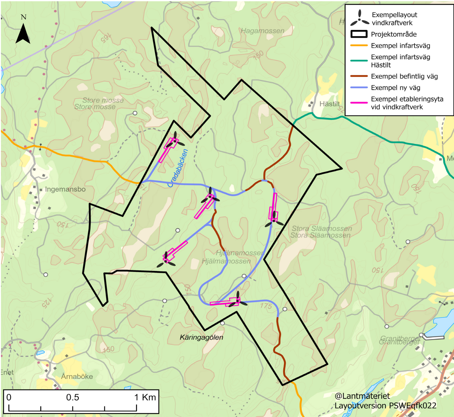
Projektområdet med en exempellayout om fem vindkraftverk med en totalhöjd på 300 meter, etableringsytor vid vindkraftverk, vägdragning och infartsvägar. Alla delar av layouten är exempel och kan komma att justeras.
